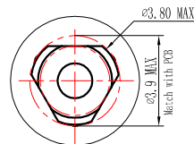
Detail C 5 : 1
