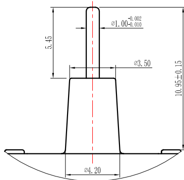
Detail A 5 : 1
