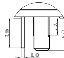
Detail D 5 : 1
