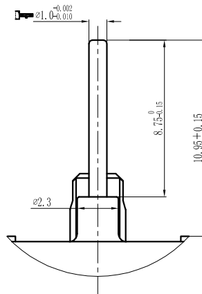
Detail A 5 : 1
