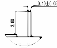
Detail B 5 : 1
