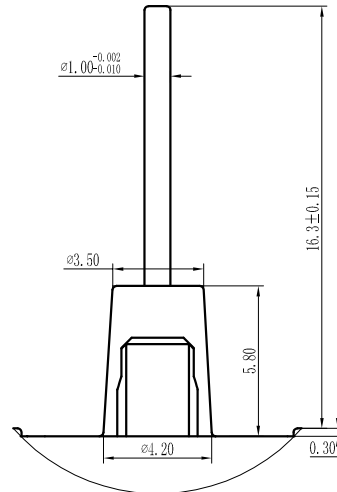
Detail A 5 : 1
