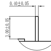
Detail B 5 : 1
