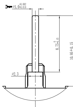
Detail A 5 : 1
